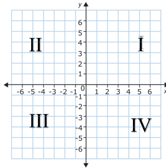
Imagen 1. Plano cartesiano
